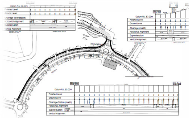
Lukisan Jajaran Jalan
